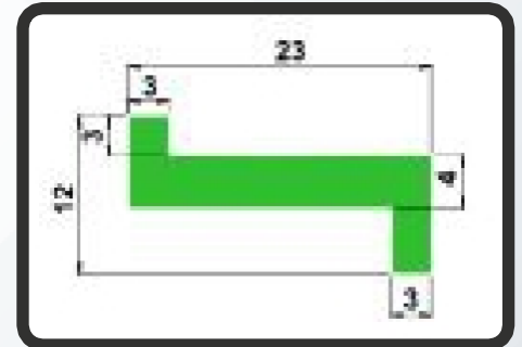
Z TYPE 23MM
